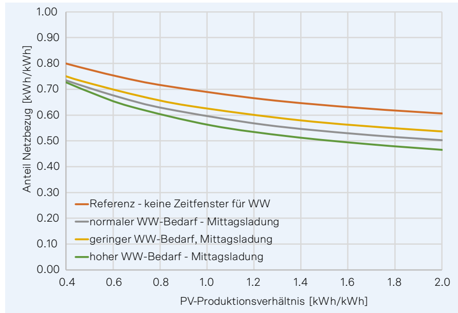
Grafik 4: Reduktion Netzstrombezug mit WP für Warmwasser
