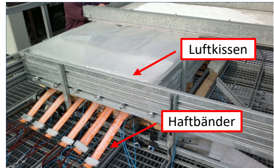
Abb. 5 Geöffnete Anlage mit Luftkissen und Haftbändern
