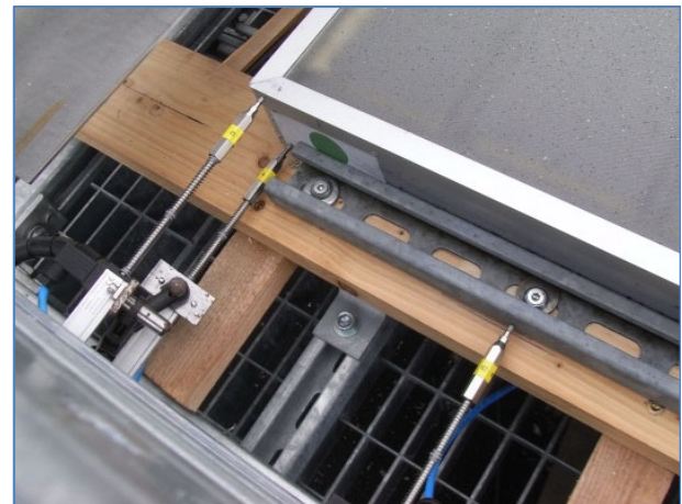
Abb.7 Distanzsensoren werden an kritischen Punkten platziert um die Verformung des Prüflings unter Last zu messen
