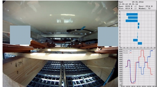
Abb.9 Weitwinkelvideokameras werden an „interessanten“ Stellen platziert und ermöglichen es den Schadenverlauf mit zu verfolgen. Gleichzeitig werden alle Kräfte und Auslenkung der Distanzsensoren angezeigt. Damit ist eine eingehende Analyse der Schwachstellen möglich. Im gezeigten Beispiel sind „vertrauliche“ Bereiche ausgegraut.
